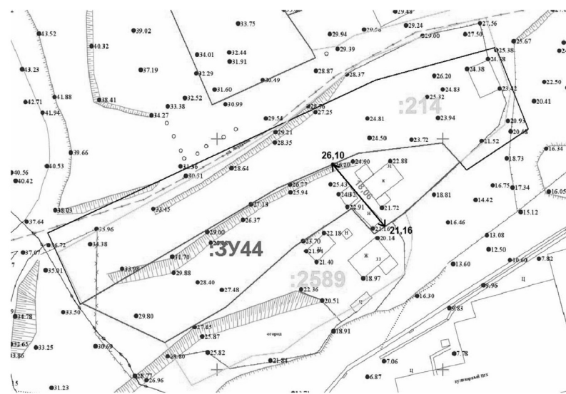
Расчет уклона на земельном участке с условным номером :ЗУ44 (чертеж 2)
